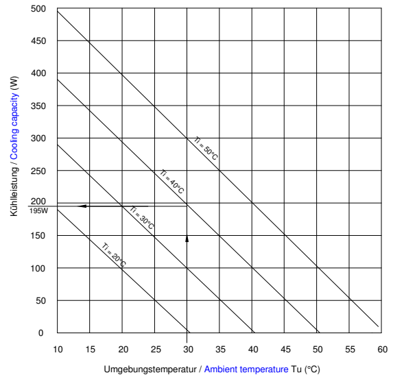
Leistungsdiagramm / Performance curve PK 100
