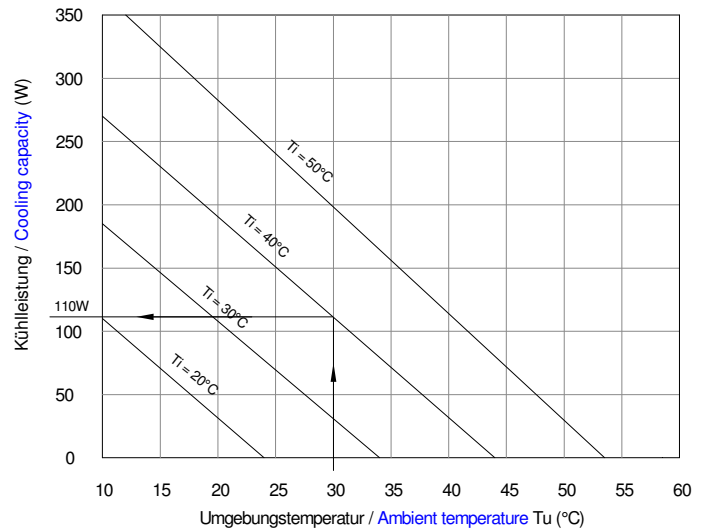
Leistungsdiagramm / Performance curve PK 30
