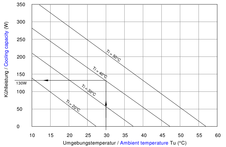
Leistungsdiagramm / Performance curve PK 50
